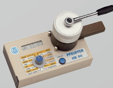
HE 50 Rutubet Ölçme Cihazı HE 50 Moisture Meter Device Влагомер HE50
