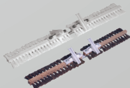
İrmik Sasör Fırçası Semolina Purifier Brush Щетка Ситовечной Машины
